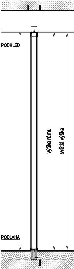
Řez V1 (1:25)
