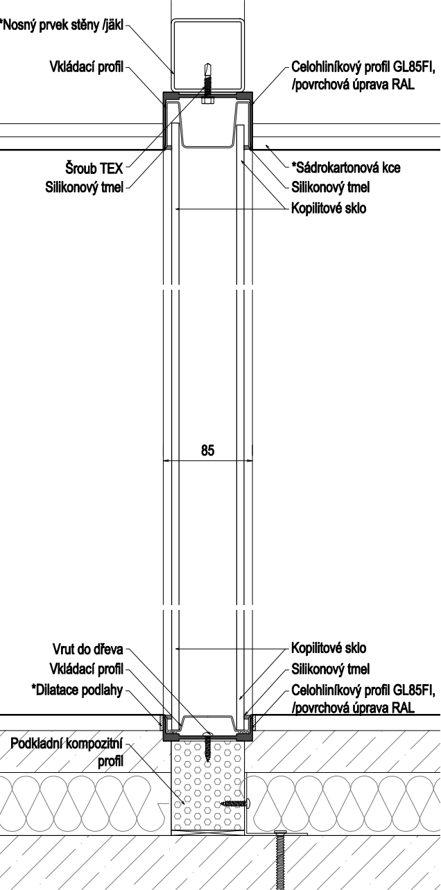
Vzorový detail_skrýtý rám
