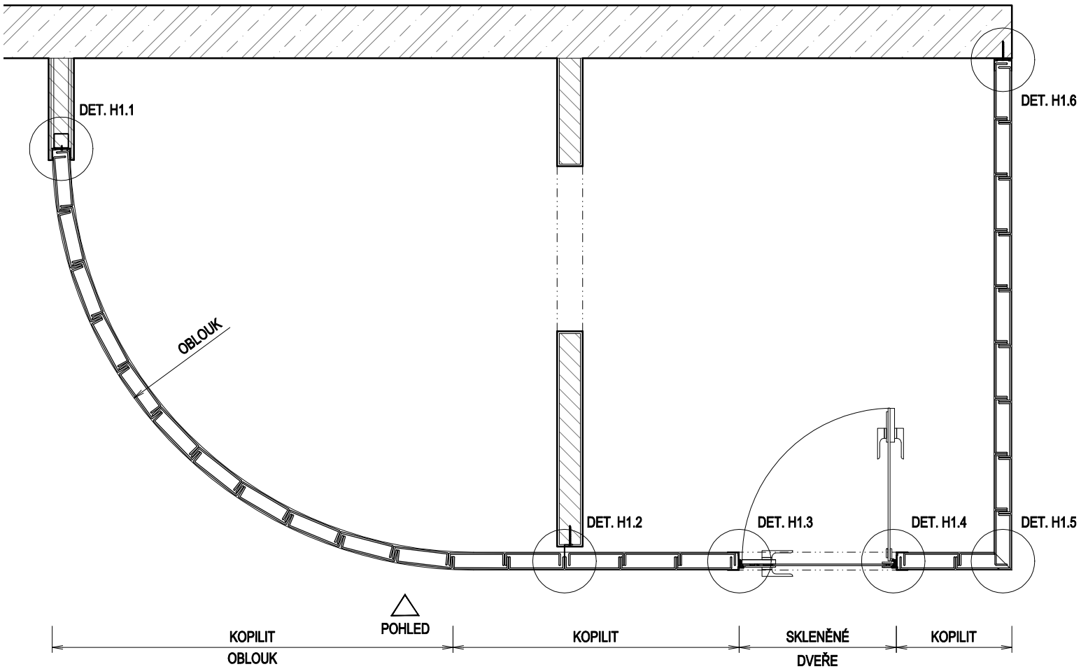
Půdorys (1:25)
