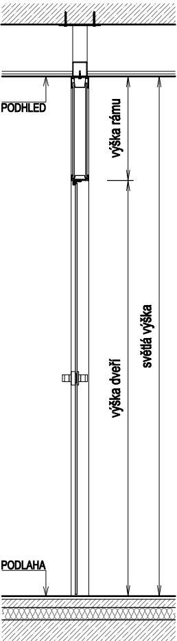
Řez V2 (1:25)
