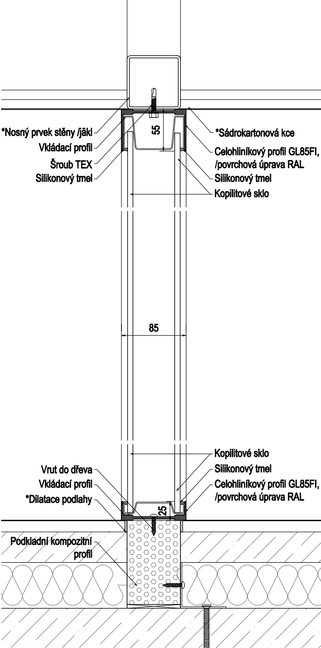
Detail V1.2 (1:5)_přiznaný rám
