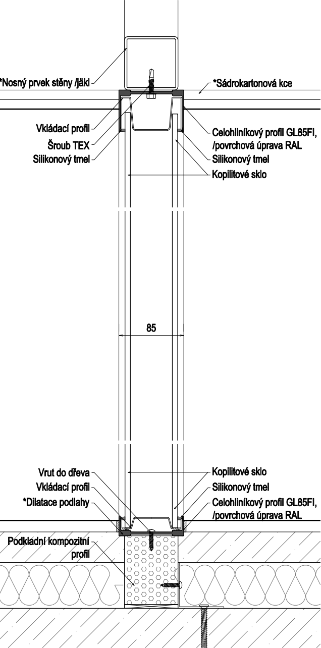
Vzorový detail_částečně přiznaný rám
